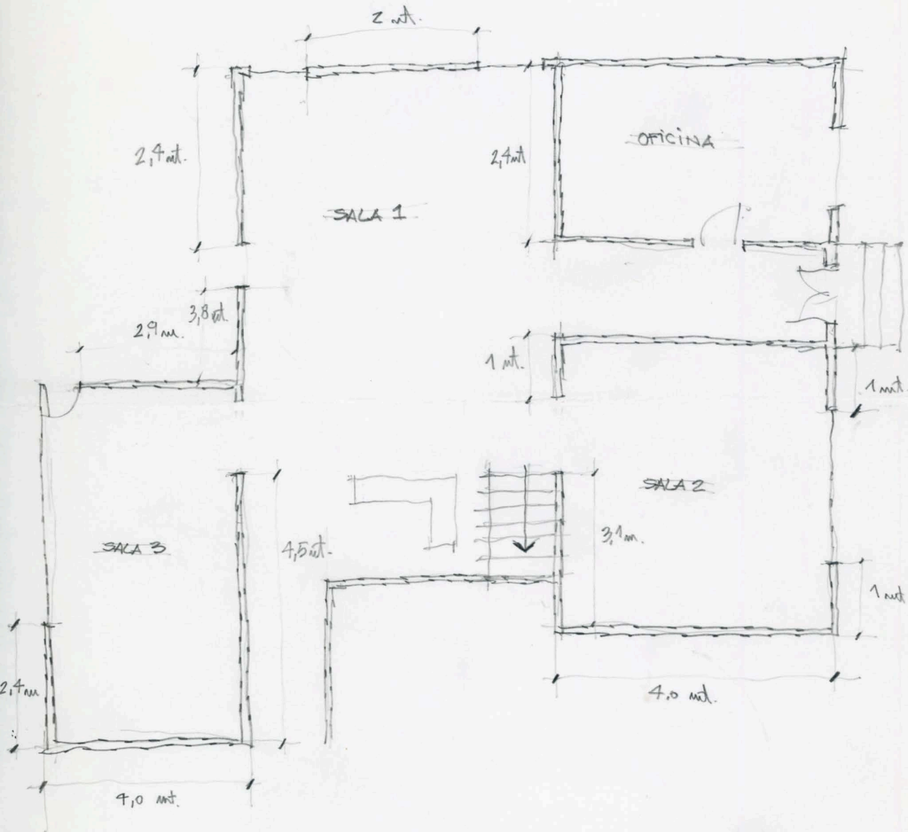
PLANTA 1er PISO ALTURA: 2.5 mt.
